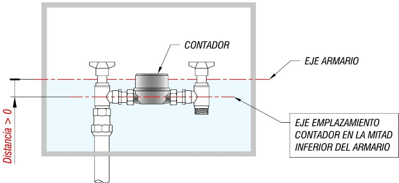
ARMARIO EN FACHADA VISTA EN ALZADO
